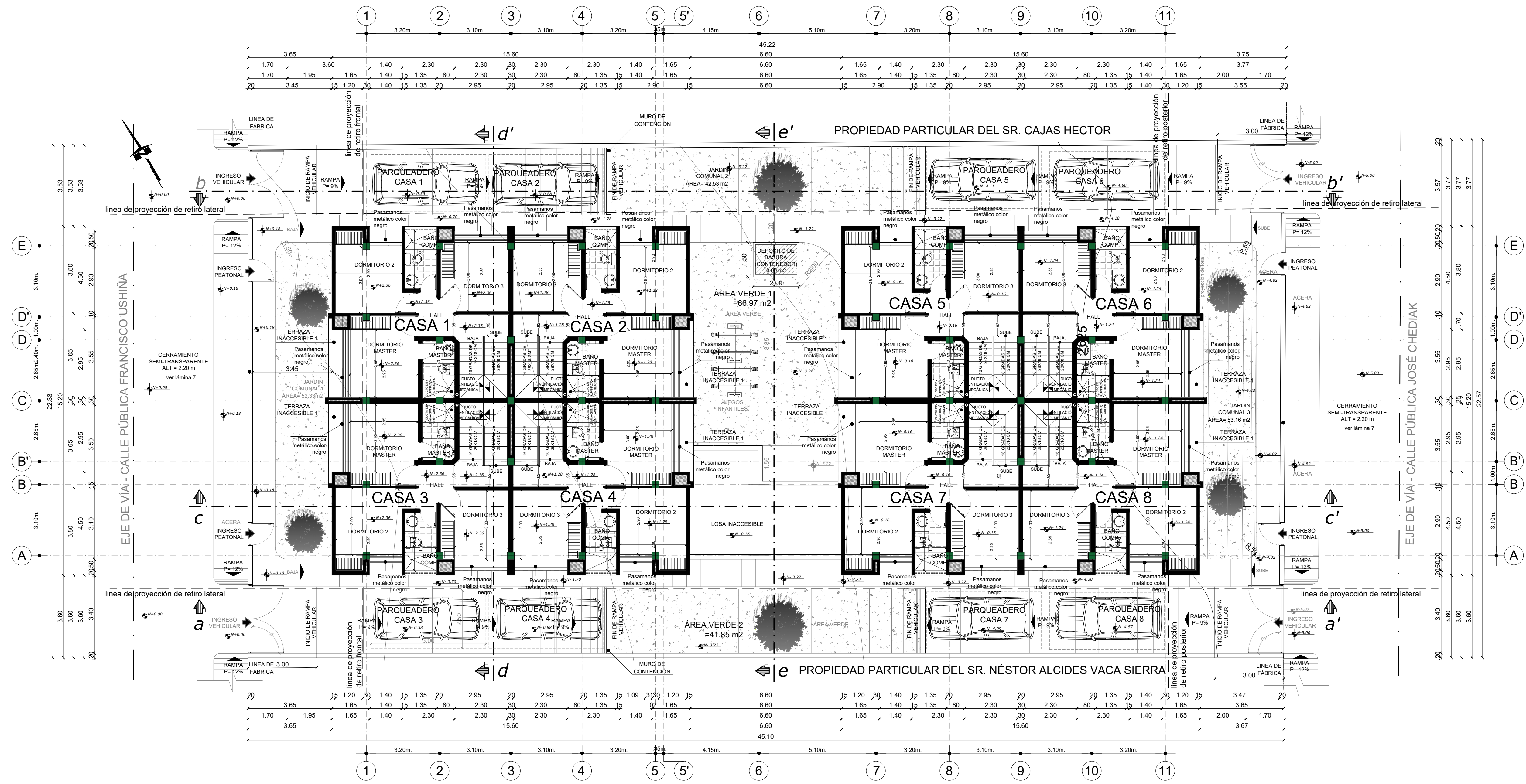
planta alta tipo escala 1:100
